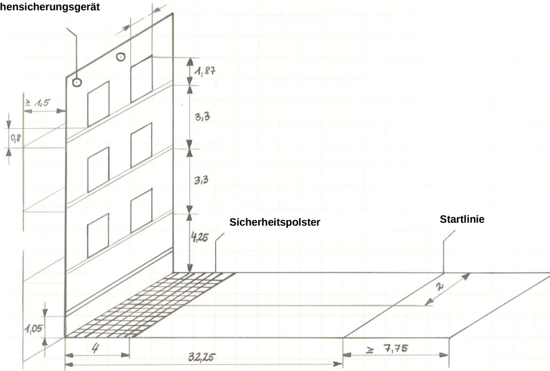
Höhensicherungsgerät
